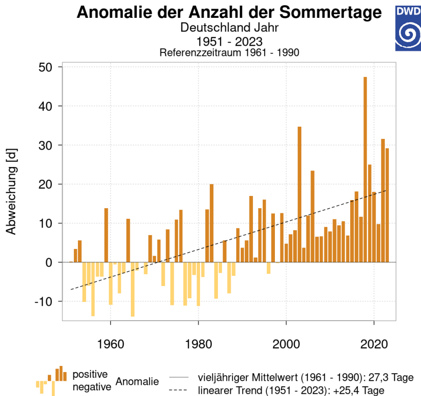
Abbildung 5: Entwicklung der Sommertage in Deutschland mit Tageshöchstwerten \geq 25^{\circ}C . Quelle: DWD
