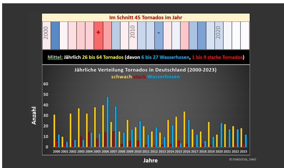
Abbildung 18: Häufigkeit Tornados in Deutschland seit 2000, siehe auch https://www.dwd.de/DE/wetter/thema_des_tages/2024/7/18.html
